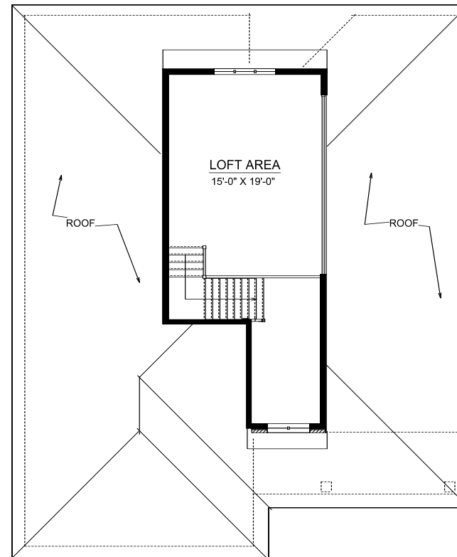
LOFT PLAN
